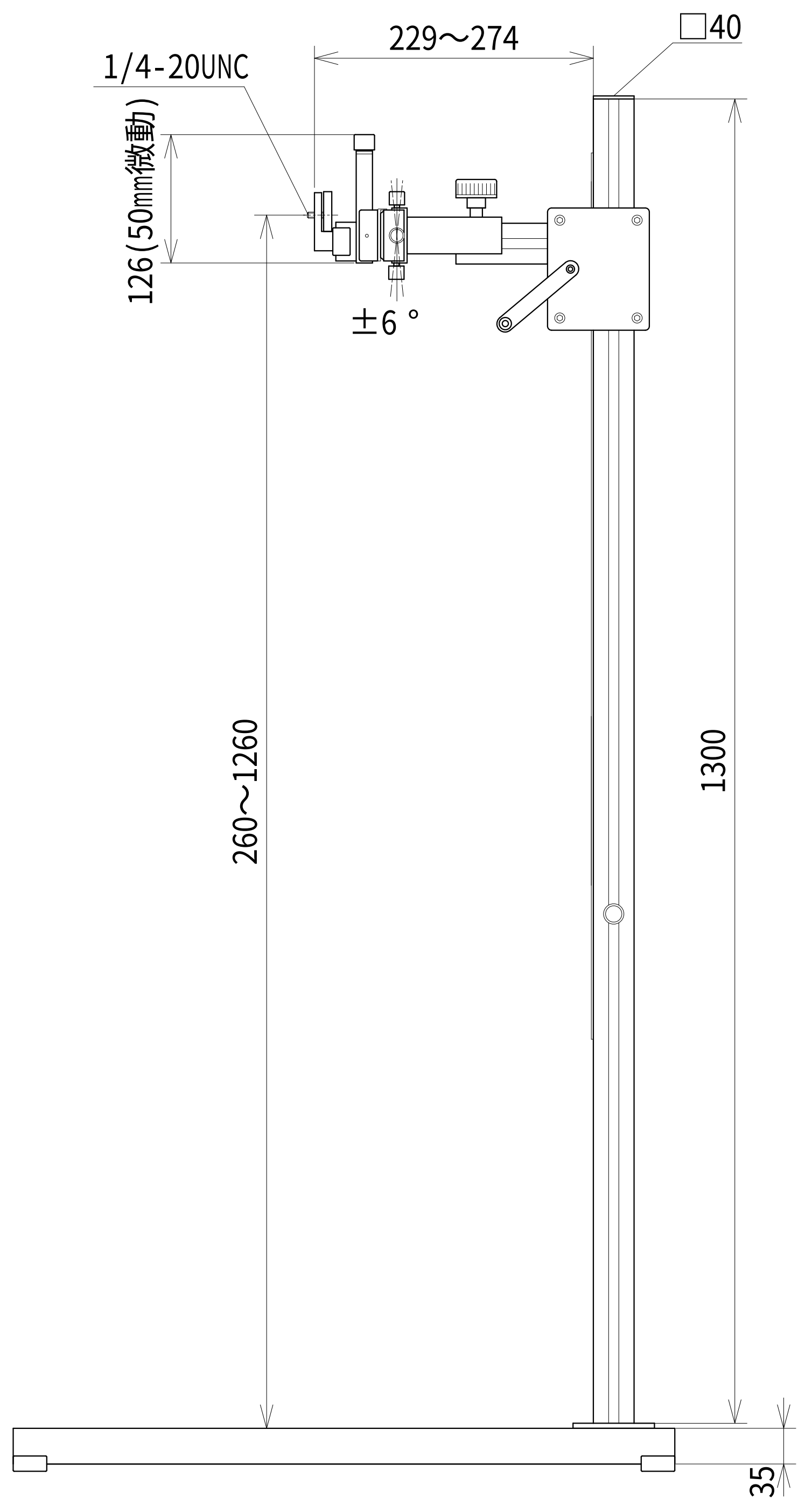
カメラスタンド1300ーR
