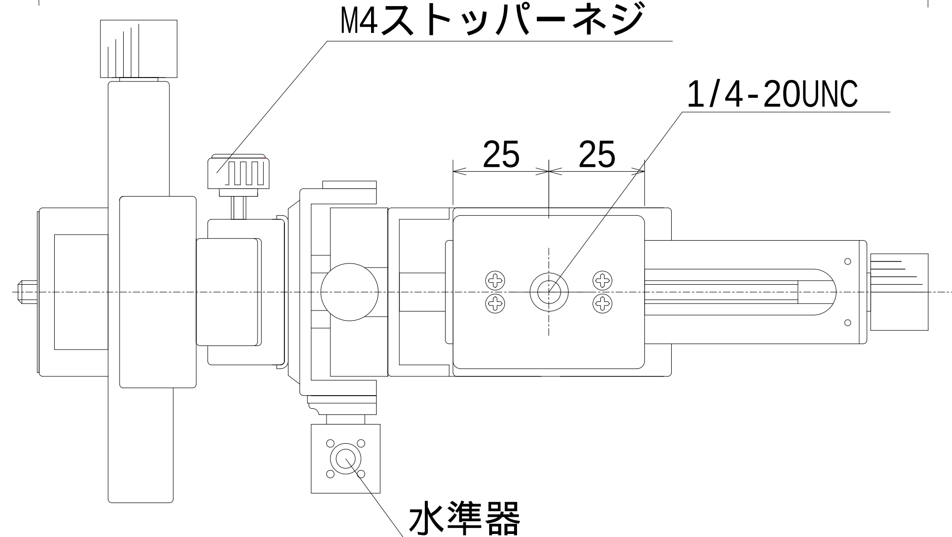
X Y Z 微動装置 - L ( ストッパー付 )
