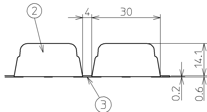
A部詳細(S=1/1)
