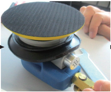
取付部が見えるように 黒いカバーを図のようにはずす
