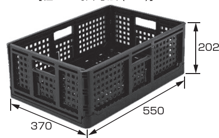
【組立て時外寸法 (mm)】
