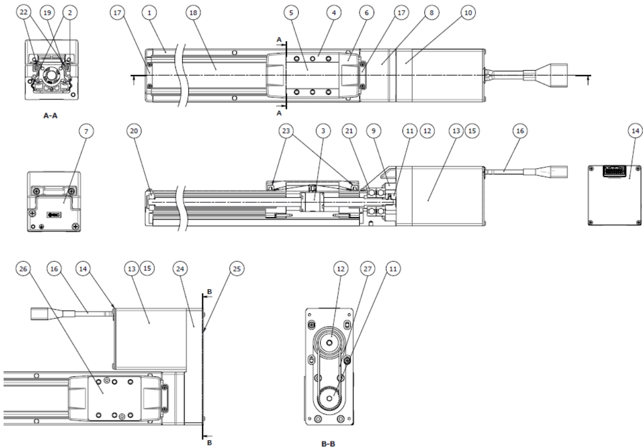
LE2FS 構成部品
