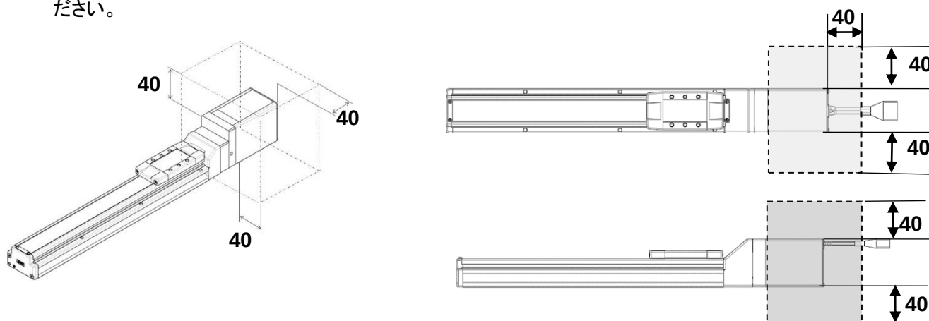
エアシリンダ設置禁止領域
