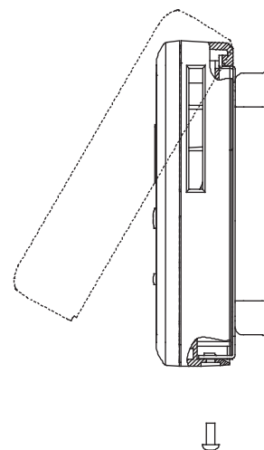
図17 取付プレートへの本体の差し込み
