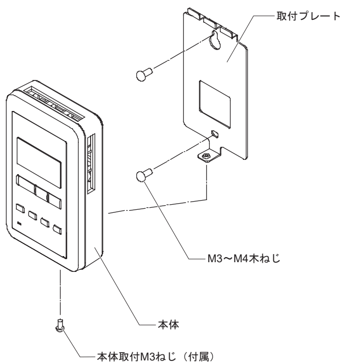
図14 壁直接取付
