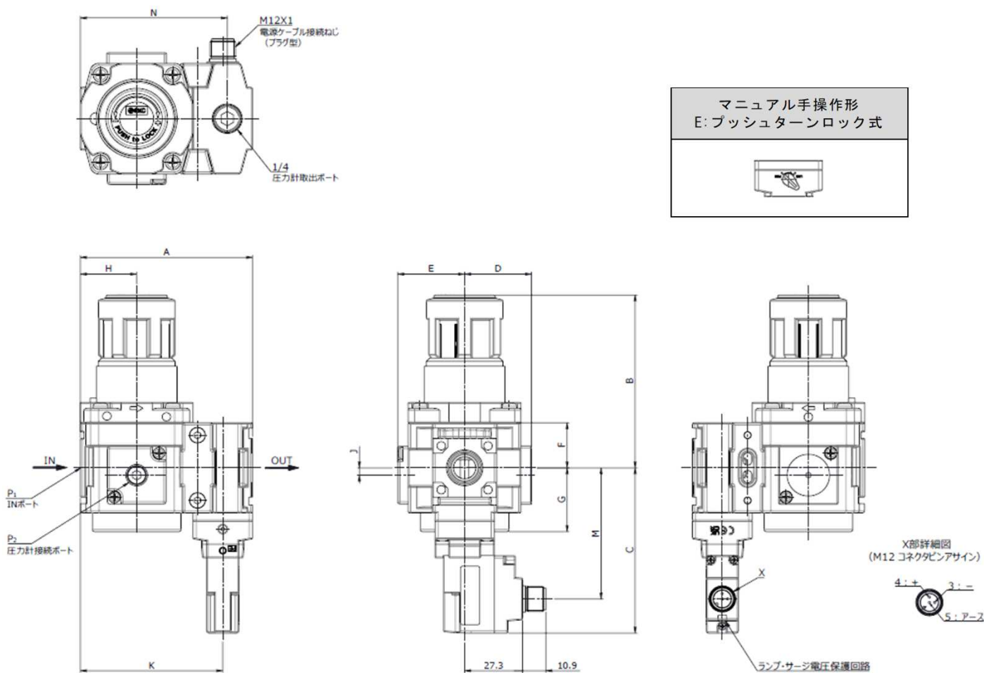
外形寸法
