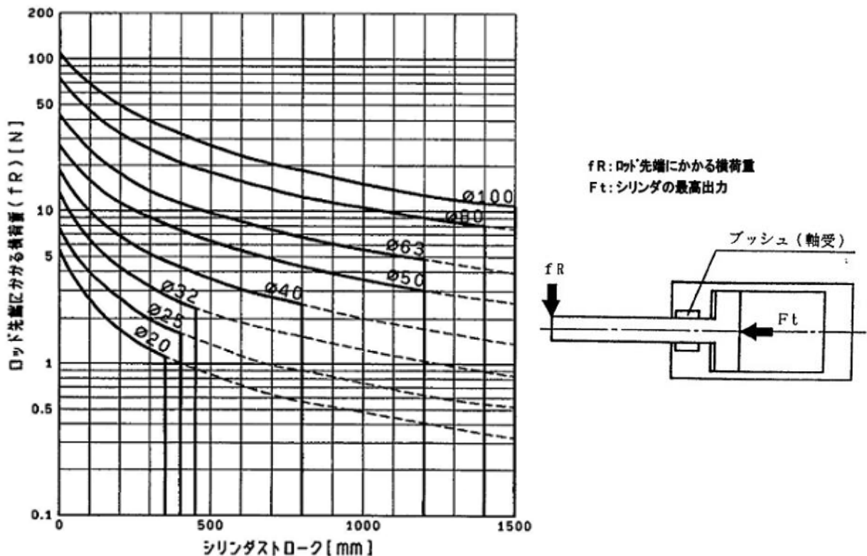
図1. ロッド先端にかかる横荷重の許容限界
