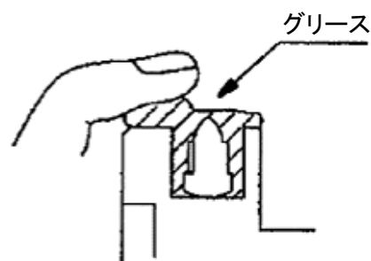
図 10. ピストンパッキン
