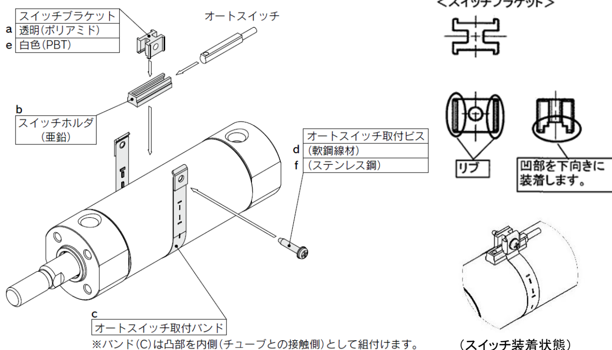
図 5. オートスイッチ取付および移動方法
