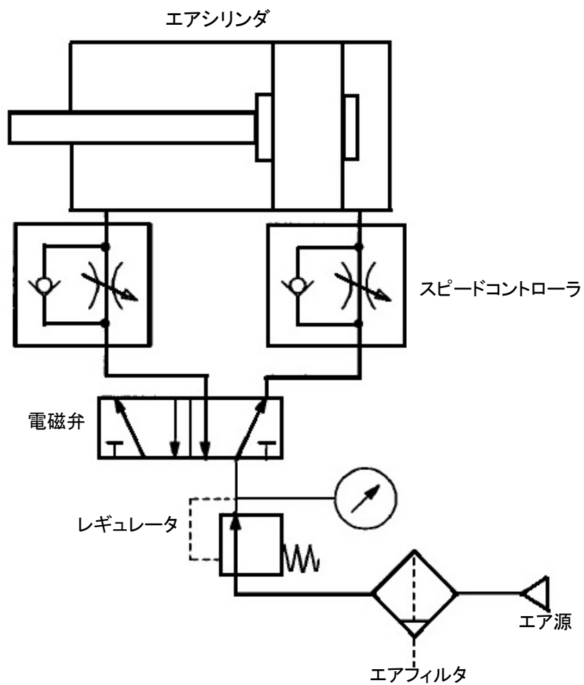
図 11. 基本回路
