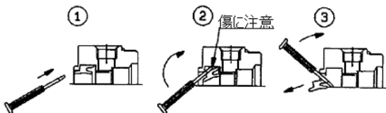
図 6. ロッドパッキン取外し方法
