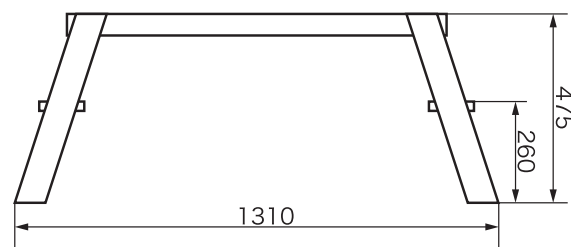
側面
