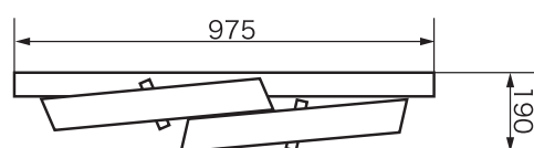
格納時
