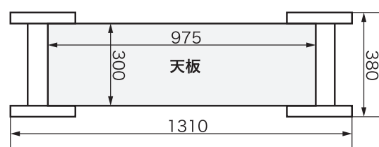
上面
