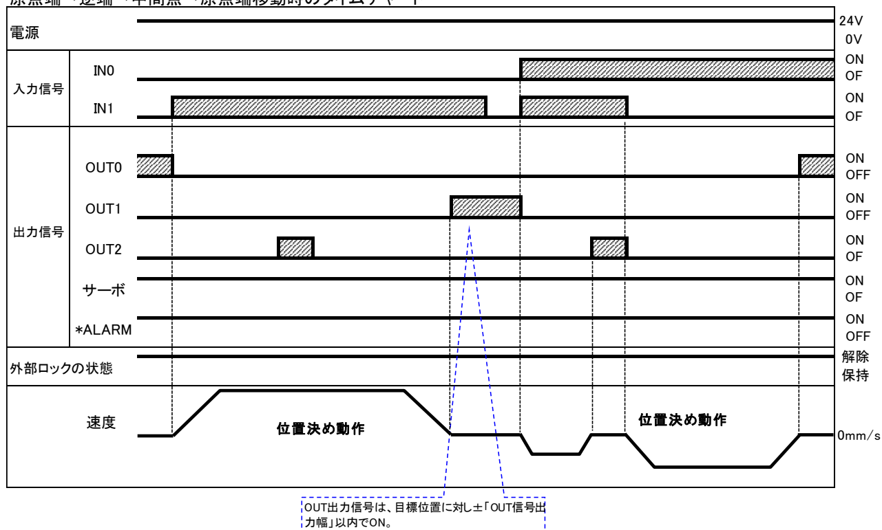
原点端→逆端→中間点→原点端移動時のタイムチャート
