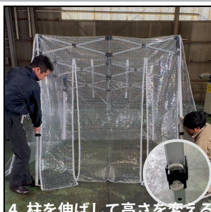
4. 柱を伸ばして高さを変える
