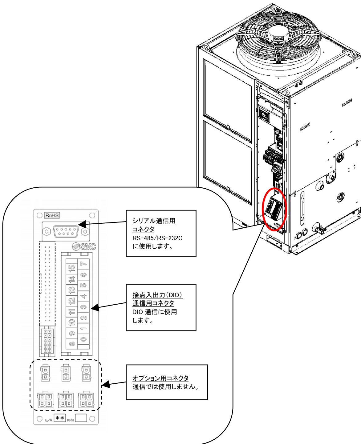
図 1.2-1 通信ポート
