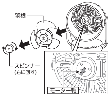
モーター軸
