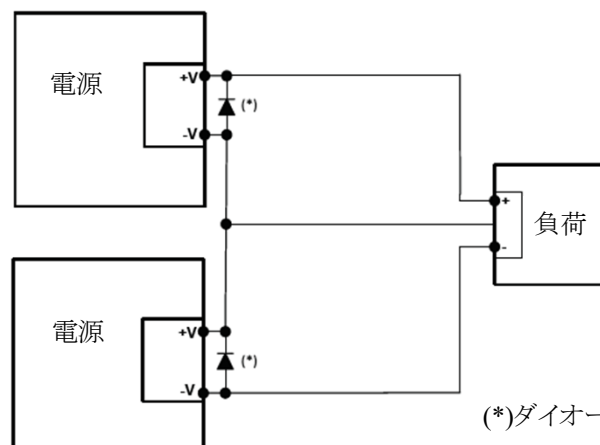
図7-10 二出力構成用の直列接続
