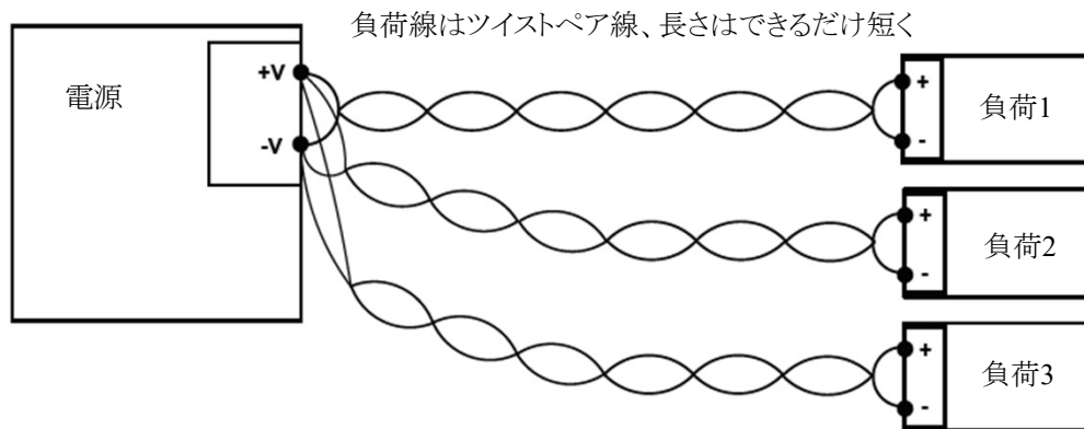
図7-3 複数の負荷への接続(ローカルセンシングの例)
