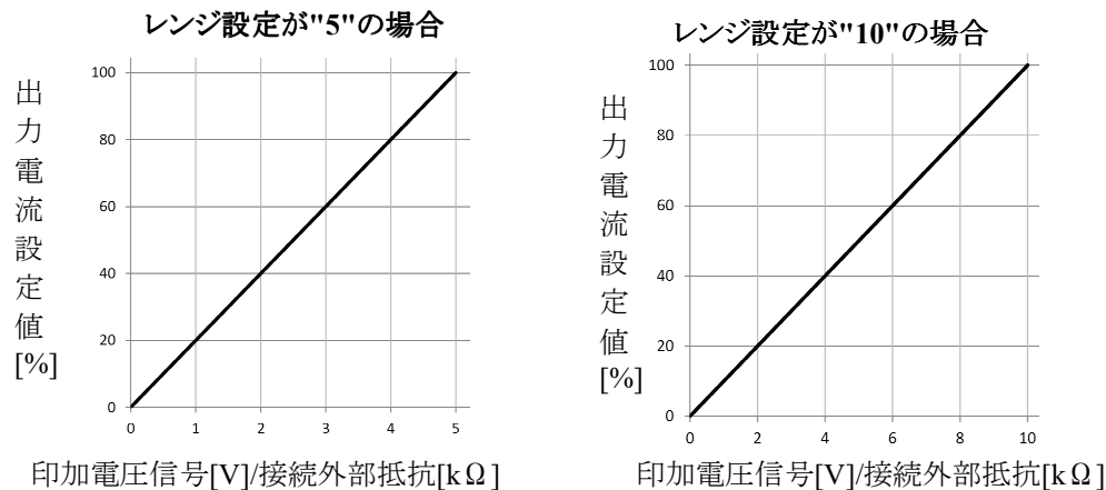
図3-6 電流プログラミング時の出力電圧設定値
