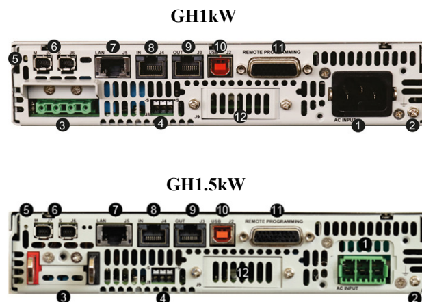
図1-9 リアパネル
