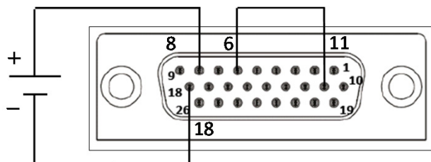
図3-4 外部電圧印加による出力電圧のリモートアナログプログラミングの接続
