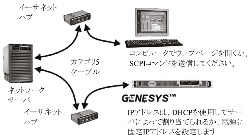
図4-6 DHCPサーバとのネットワーク
