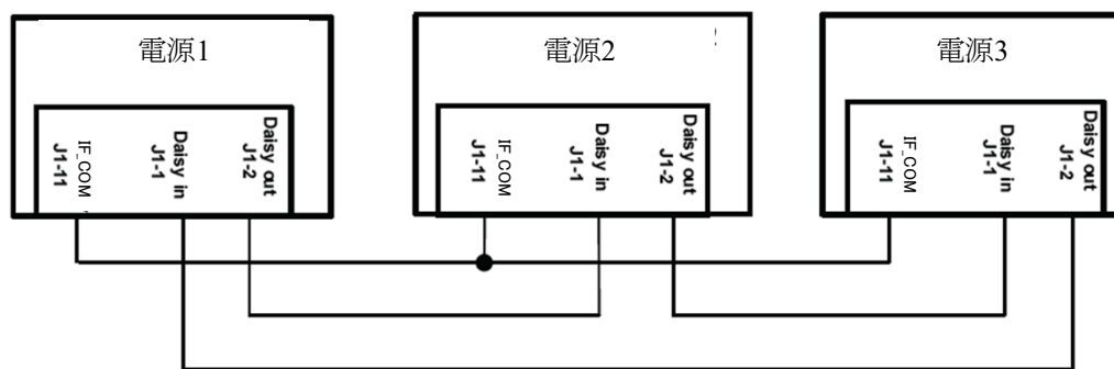
図7-13 デイジーチェーン接続
