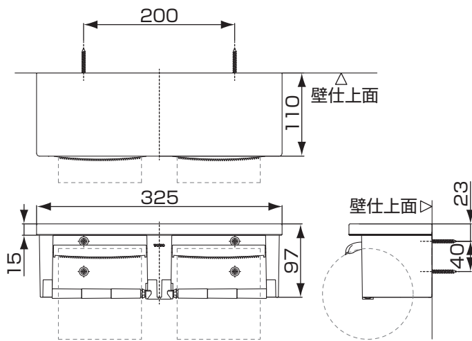
YH651型 芯なしペーパー対応
