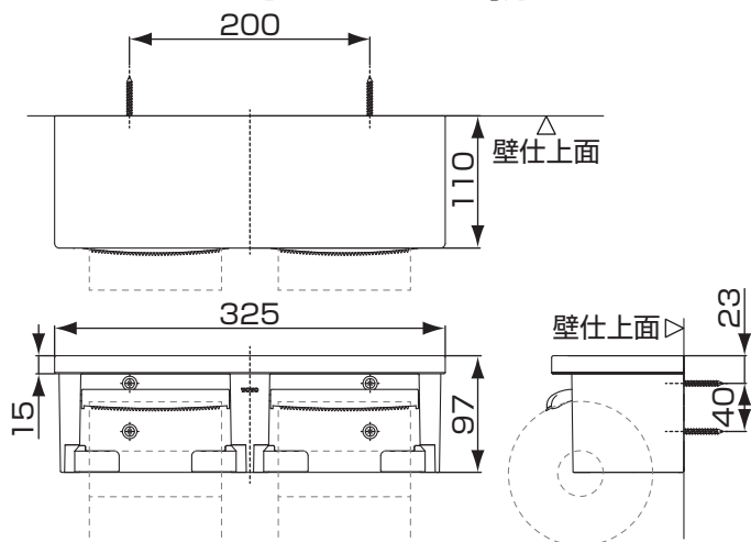
YH650型 芯ありペーパー対応
