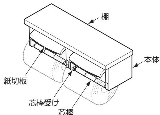
YH651型 芯なしペーパー対応
