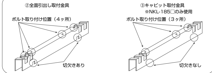
②全面引出し取付金具と③キャビネット取付金具の形状詳細図
