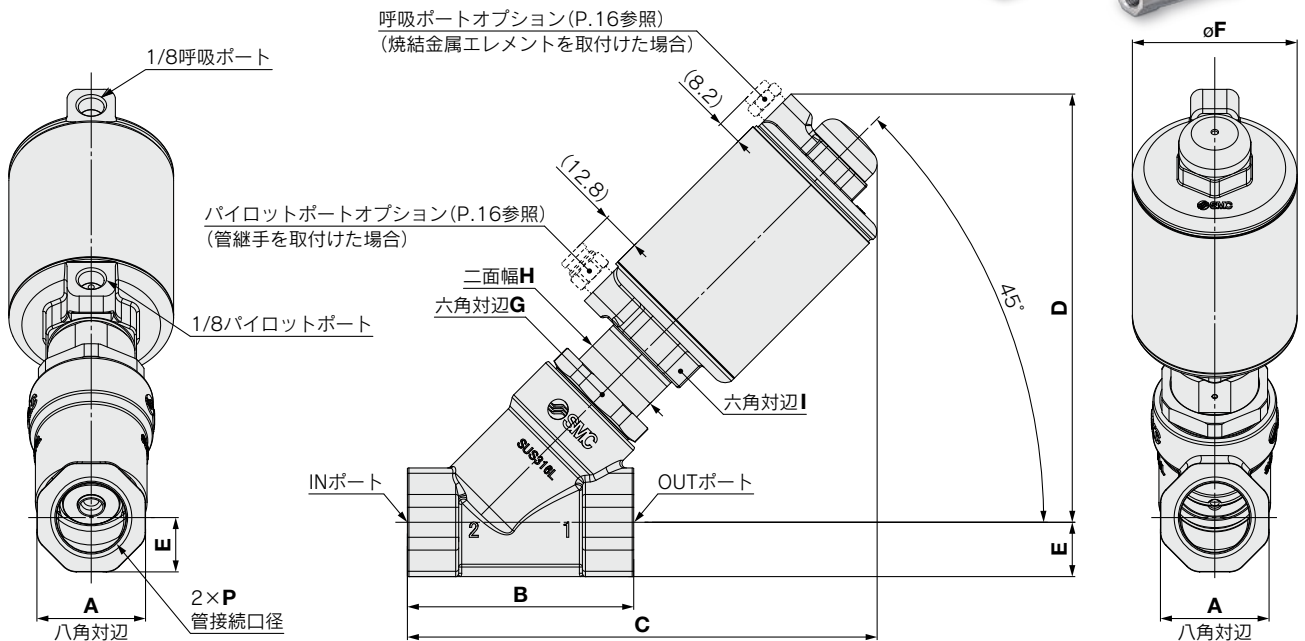
寸法表
