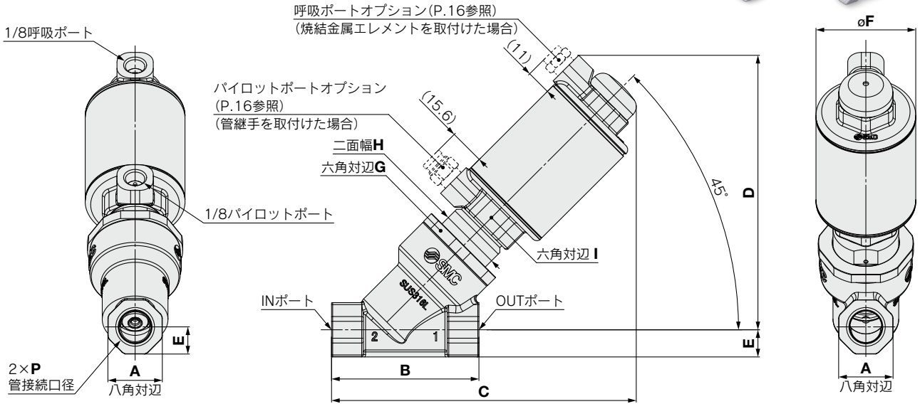
寸法表
