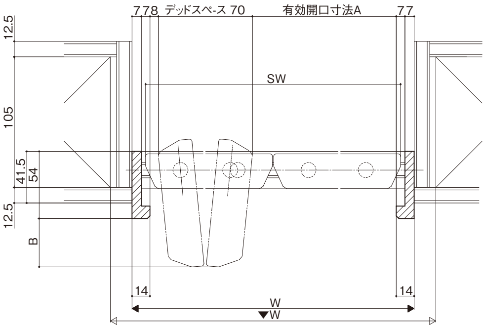
横断面図
