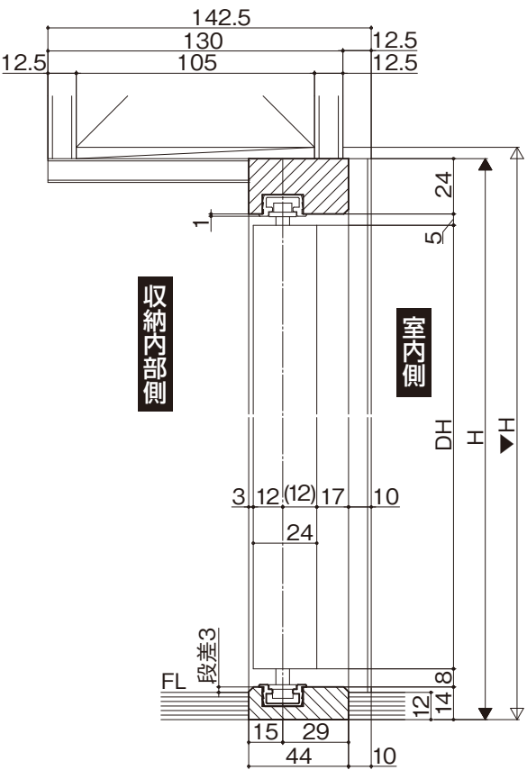
縦断面図
