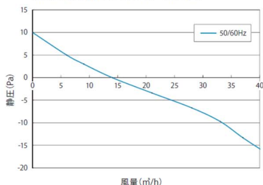
静圧-風量特性グラフ(P-Q曲線)
