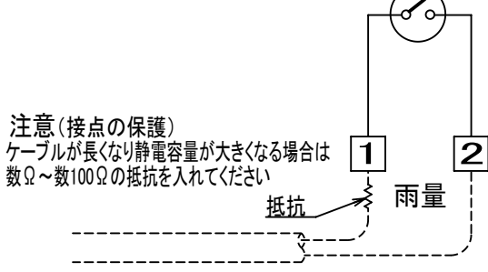
雨量接点配線例
