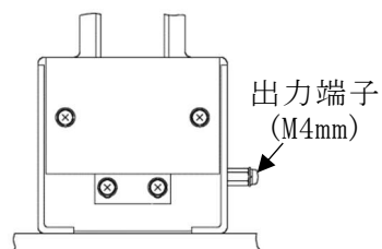
図5：接点出力端子1回路(W無し)
