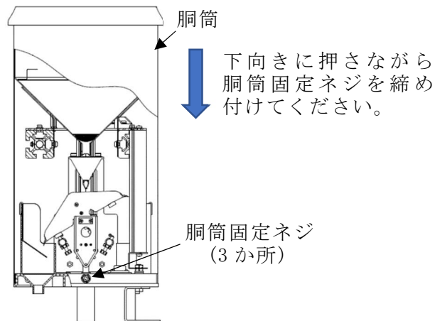
図8：胴筒の固定(ヒーター付きの場合)
