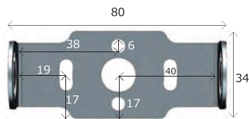
・カメラ設置ブラケット寸法(mm)
