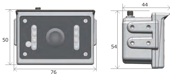
・カメラ本体寸法(mm)
