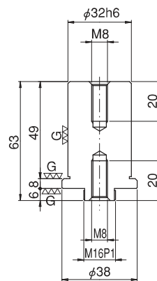
シャック \phi 32 mm
