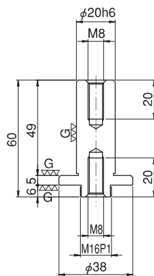
シャック \phi 20 mm
