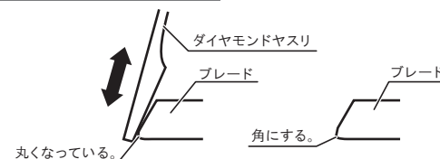
図1 (ブレード側面部の断面図)
