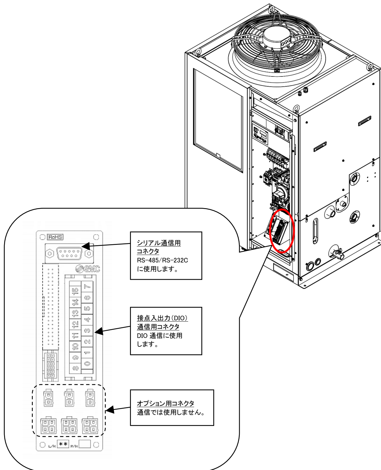
図 1.2-1 通信ポート
