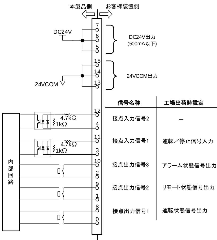
図 2.3-1 接点入出力回路
