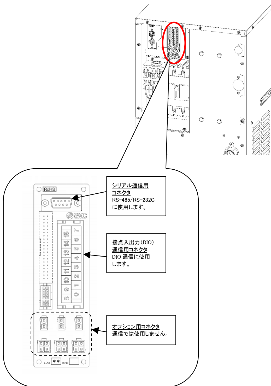
図 1.2-1 通信ポート
