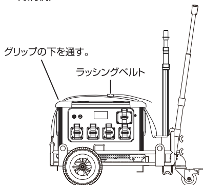
〈取付例〉
