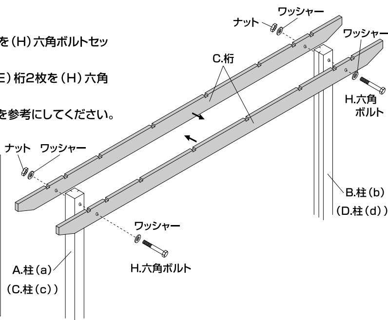
D.柱(d)
