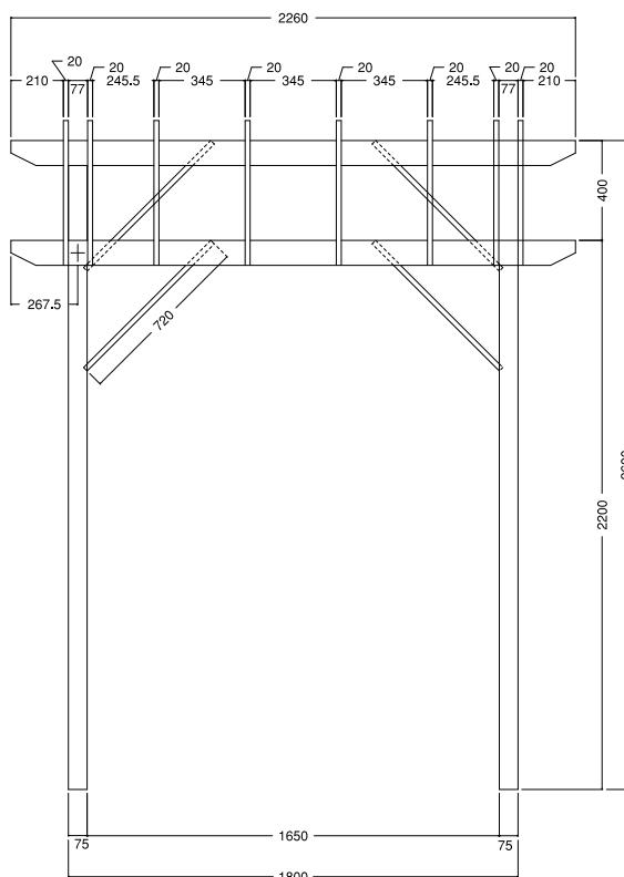
〈正面図〉
