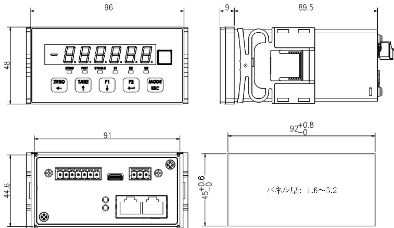
外形寸法図
