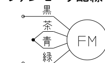
OC-12(S)-A200 ファンモータ配線
