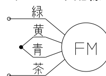
ファンモータ配線
