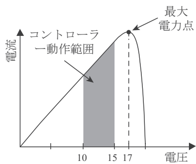
出力電力(12Vシステム)
