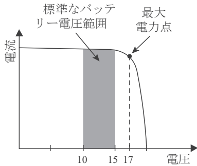
電流vs.電圧(12Vシステム)
