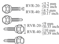
セルフタッピングボルト
