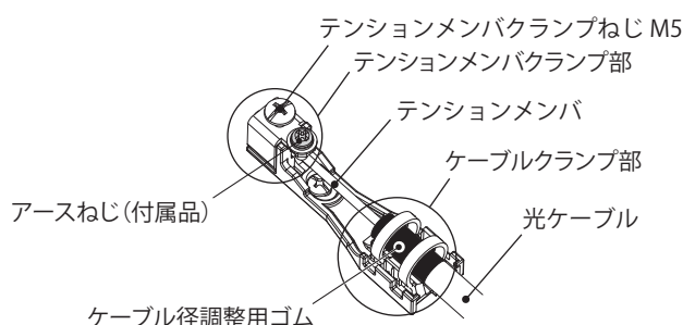
図1 光ケーブル固定
