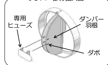
ダンパー部分拡大図
