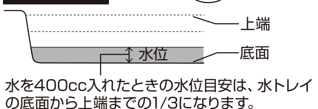
水トレイの断面図
