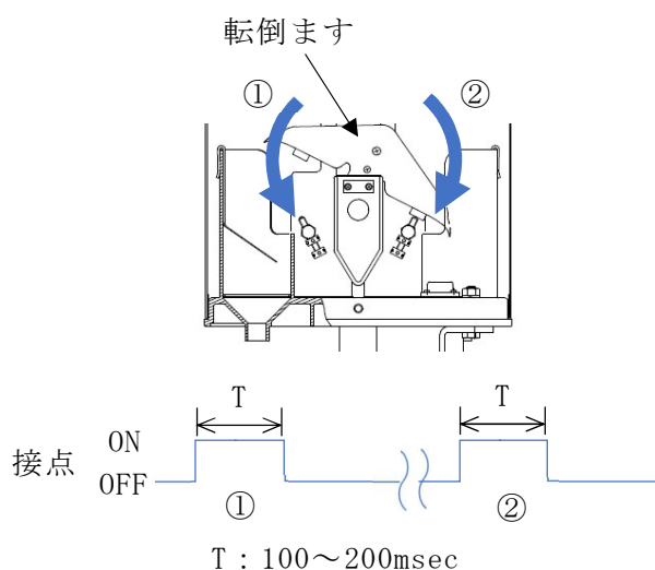
図2：接点タイミング図
