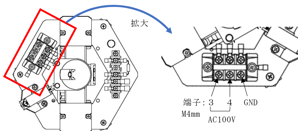
図 7：ヒーターユニット上面図
