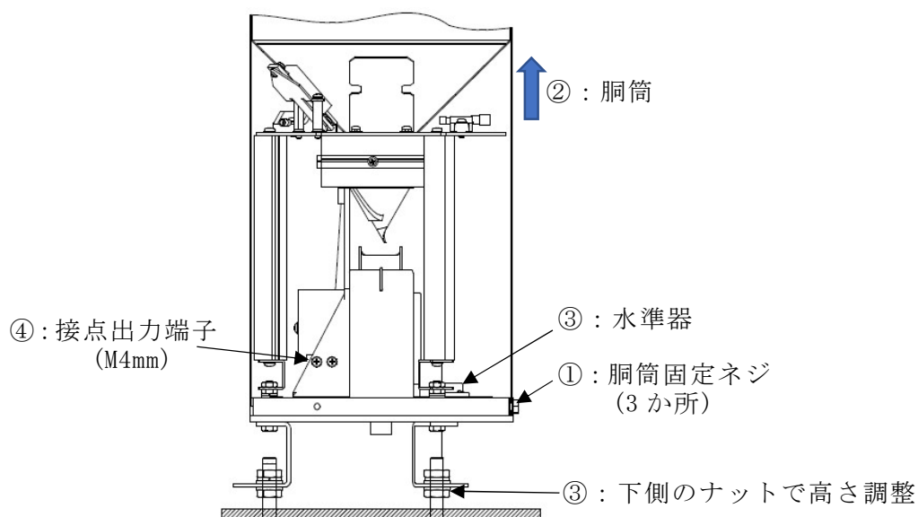
図4：構造図(ヒーター有り)
