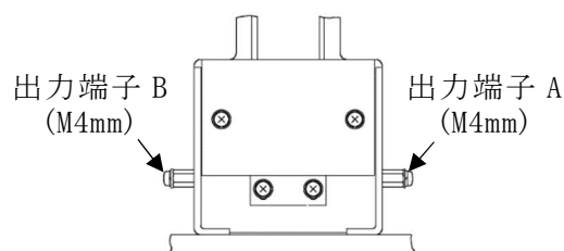
図6：接点出力端子2回路(W付き)
