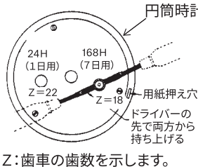
図4. 歯車の取り外し
