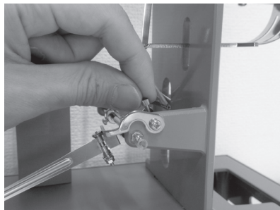
図10. 微調整ネジ (湿度)
