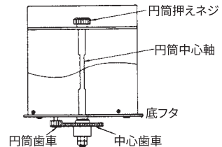
図8. 円筒の取り付け
