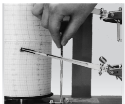
14.ペン押え金具を上を持ち上げて外す。
