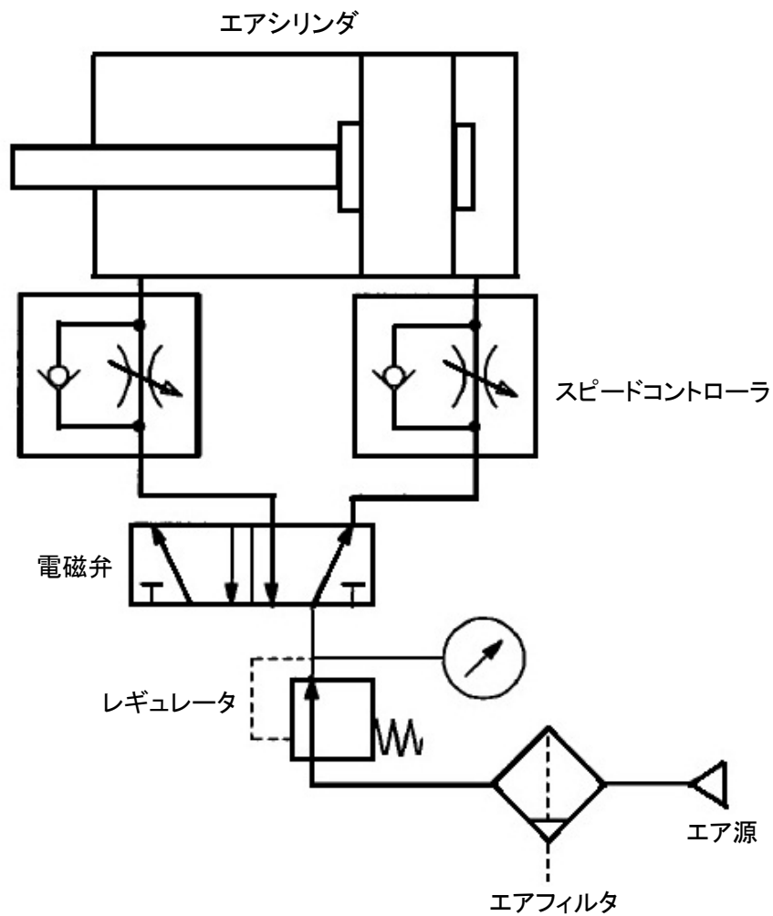
図 4. 基本回路
