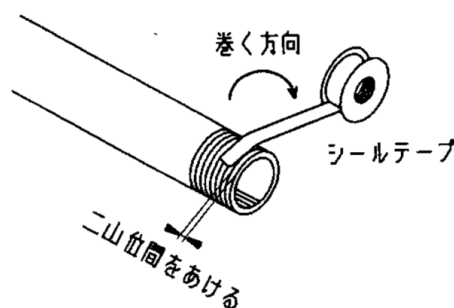
図 2. シールテープの巻き方
