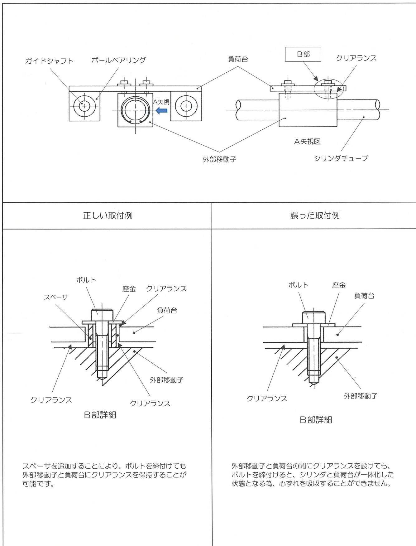
図8 シリンダと負荷との心ずれが吸収できない取付例②
