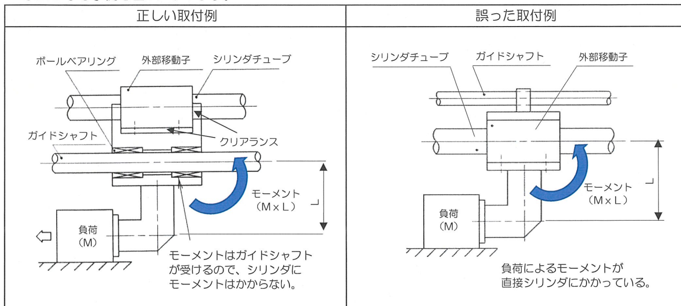
図6 過大なモーメントがかかる取付例
