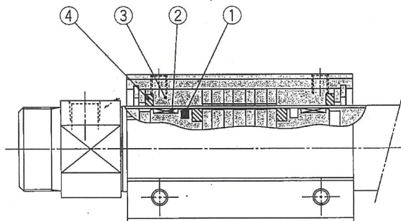
CY3B15~40-□Z
