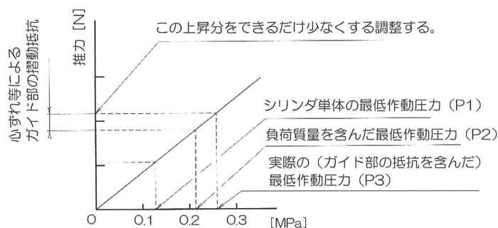
図10 最低作動圧力
