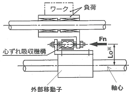
図11 駆動力とモーメント
