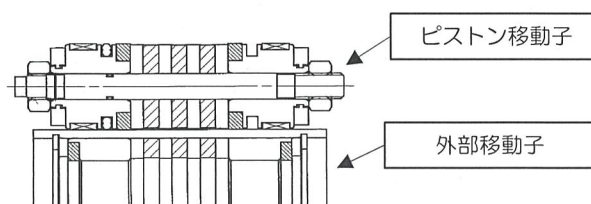
図17 正しい組み合わせ
