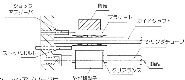
図14 ストローク端のモーメント対策例
