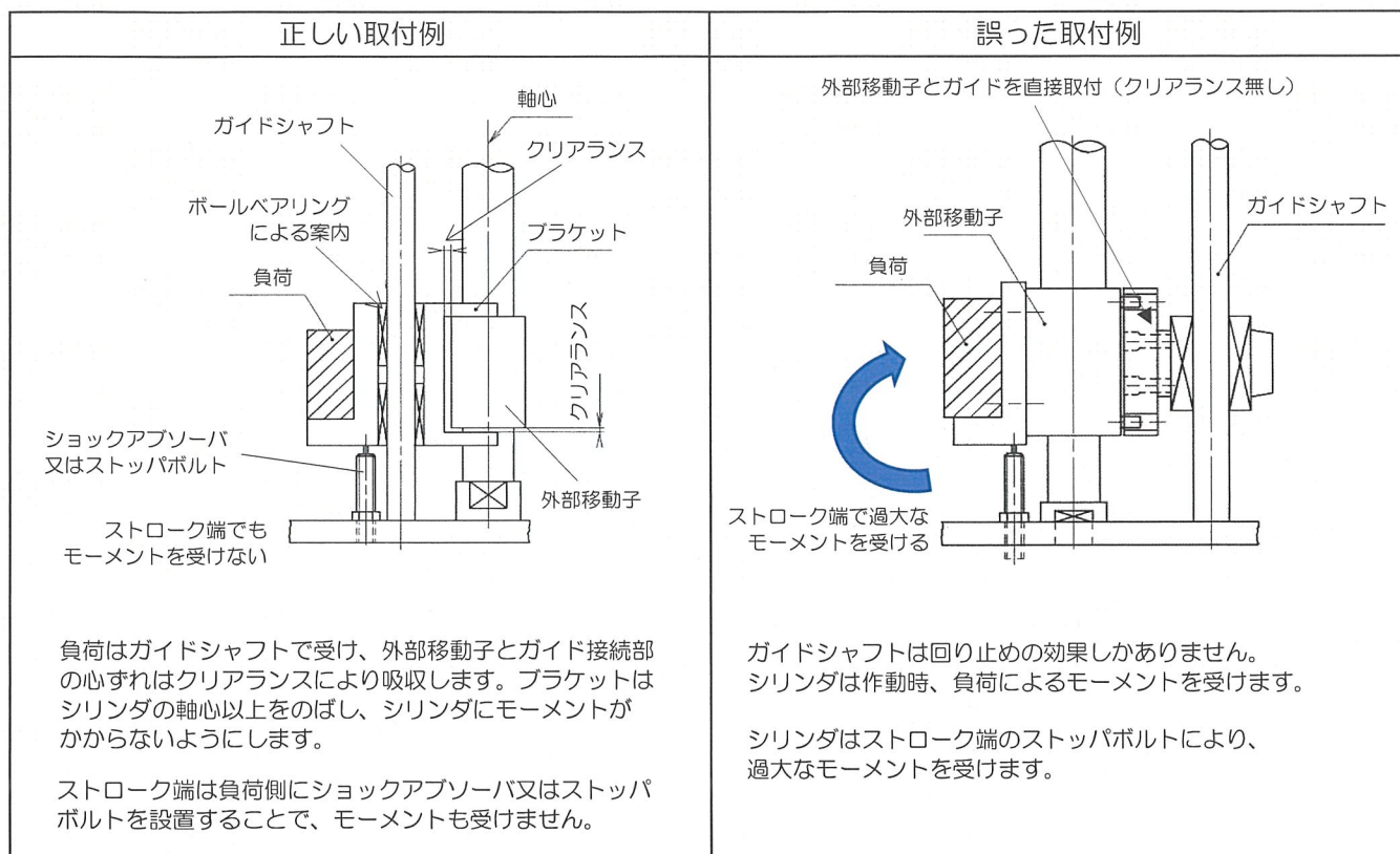
図9 シリンダと負荷との心ずれが吸収できない取付例③
