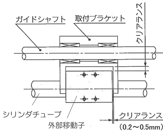
図5 負荷との接続
