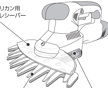
芝生バリカン用 櫛刃付刈込高 調整フレーム
