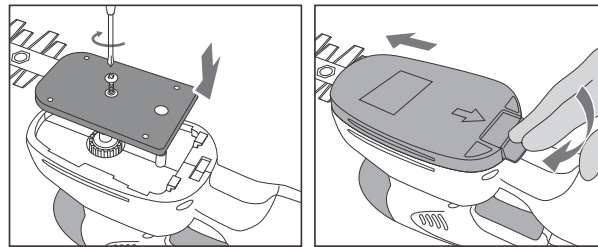
コードレス ヘッジトリマー替刃 YHK-300 JAN コード :4983771261930
