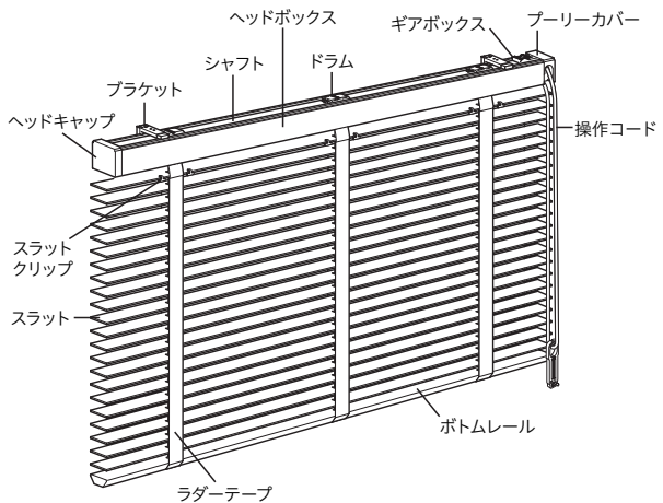
全体図
