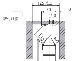
カーテンボックス納まり図 (mm)
