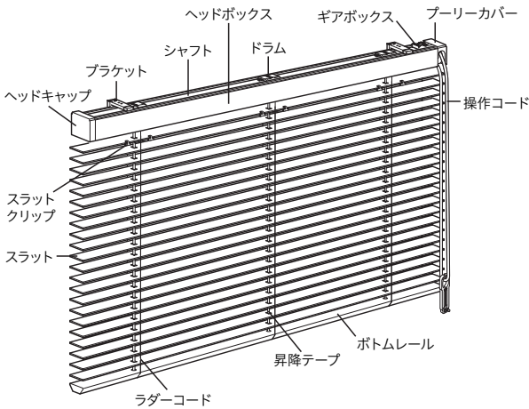
全体図
