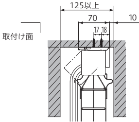
カーテンボックス納まり図 (mm)
