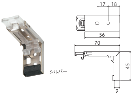
ブラケット (mm)
