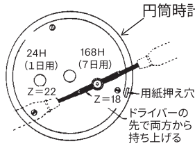
図4. 歯車の取り外し
