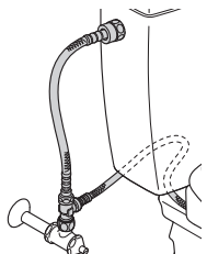
取付完成図
