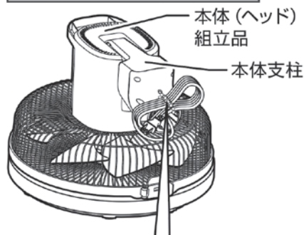
ベース表面に組立品をのせた状態
