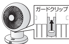
⑥▲を■に合わせてガードをはめ込み、▲を■に合わせるガードクリップを閉じ、ガードを固定する
