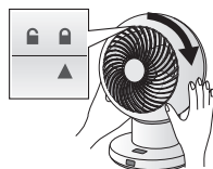
⑥▲を■に合わせてガードをはめ込み、▲を■に合わせるガードクリップを閉じ、ガードを固定する
