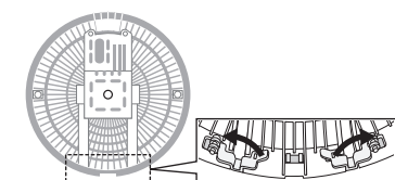
①ガードクリップ(内側2箇所)を開く
