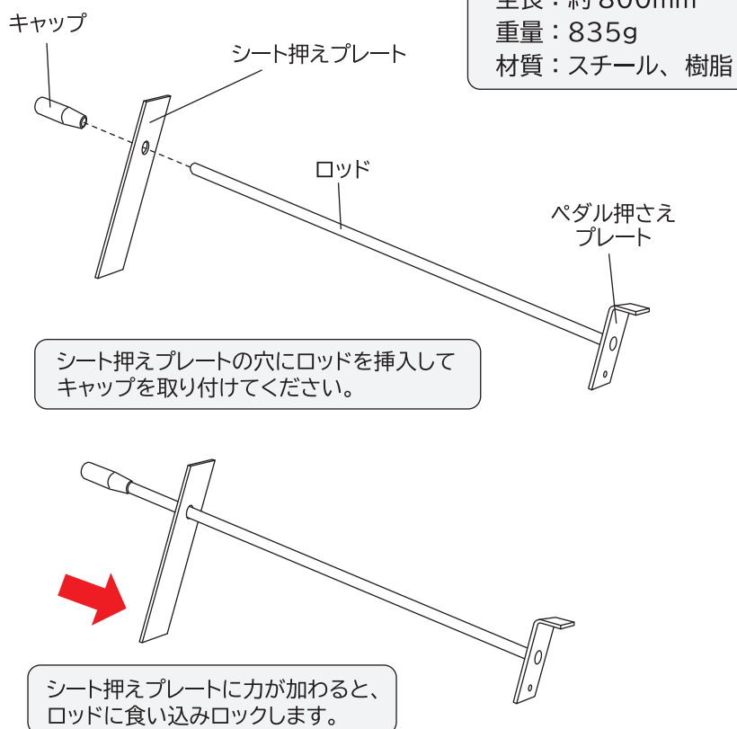
装着図 (シート付近)
