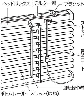
ブラケット
