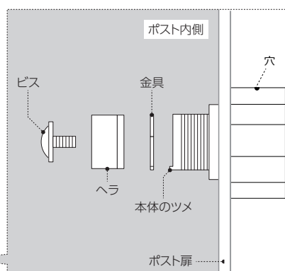
ヘラの向き
