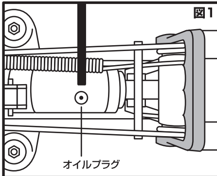
リフトアームを最降下させ、カバーを開き、平らな場所でオイルプラグを外してください。
