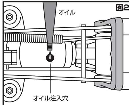
ジャッキオイルを少量ずつ注入してください。オイルの補充が終わりましたら、エア抜きを行ってください。
