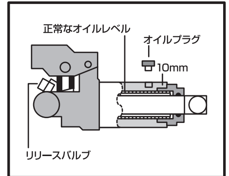
オイルをバルブの穴より10mmくらいまで補充してください。
