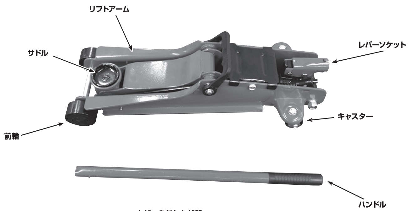
カバーを外した状態
