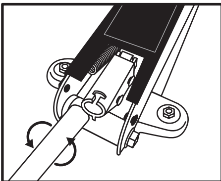
レバーを左に回してリリースバルブをゆるめてください。(2~3回転)
