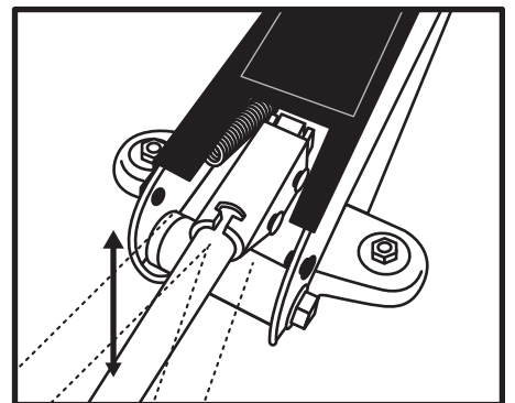
レバーをソケットに差し込み、上下いっぱいにはポンプ操作してください。(すばやく5~6回)その後、オイルプラグをしっかりと締め、カバーを閉じてください。
